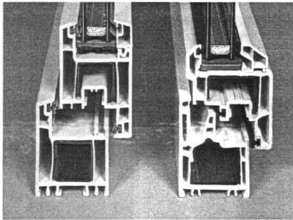
DECEUNINCK MONDIAL 20000
