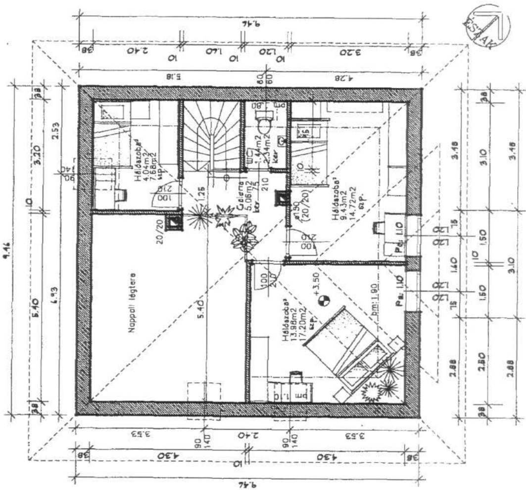
Tetőtéri Alaprajz M=1:100
