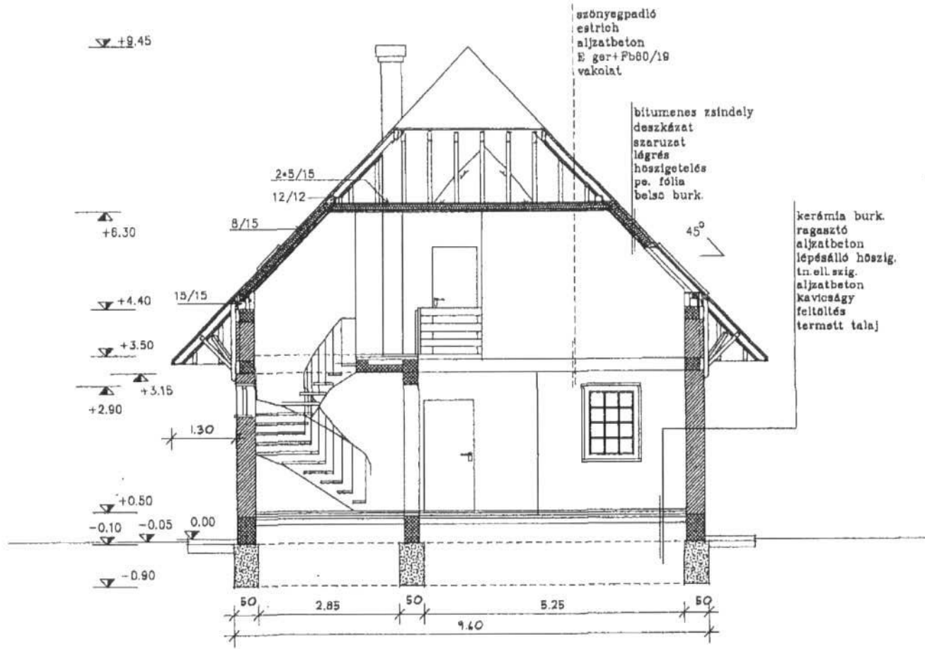
A - A Metszet M=1:100
